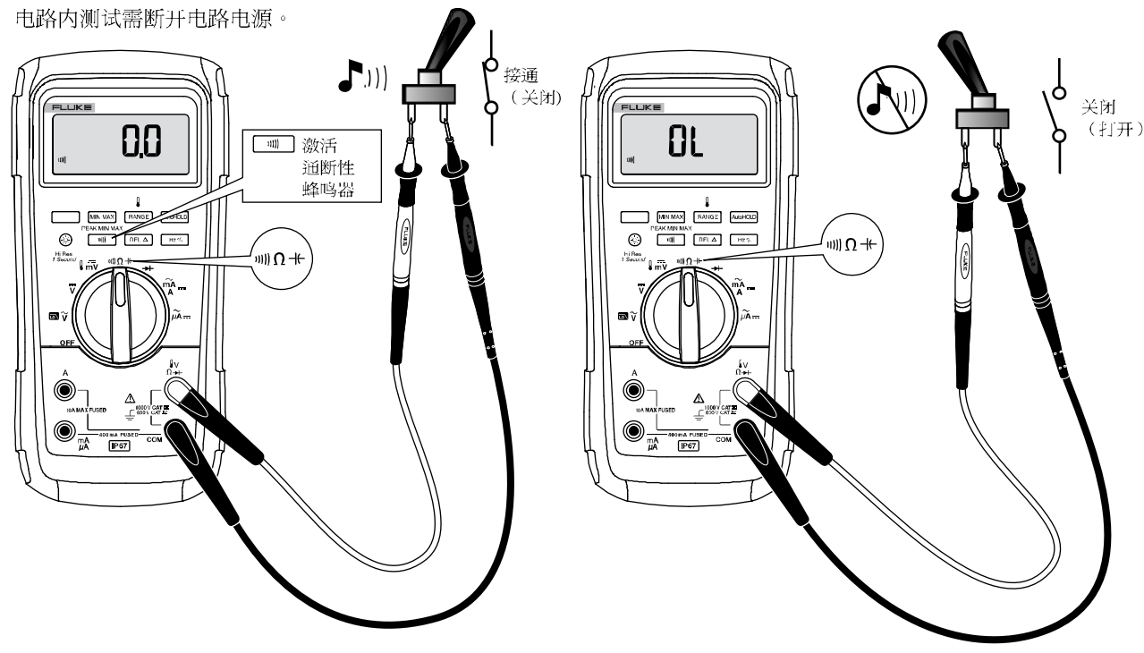
图 4.通断性测试
