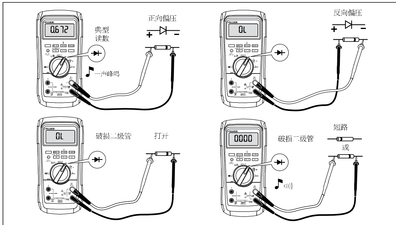
图 7.二极管测试
