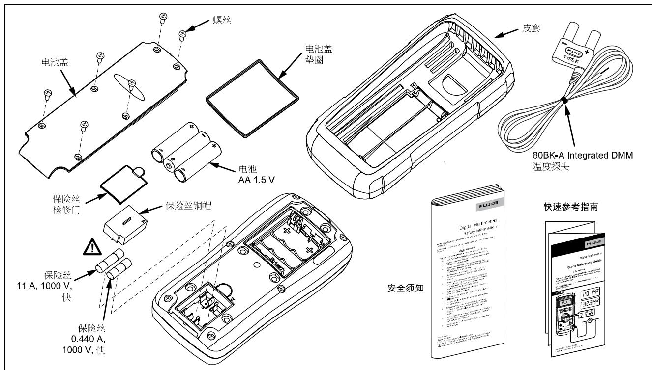
图 12.可换部件
