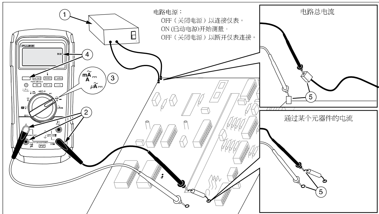
图 8.电流测量
