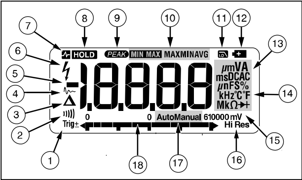
图 1.显示屏功能
